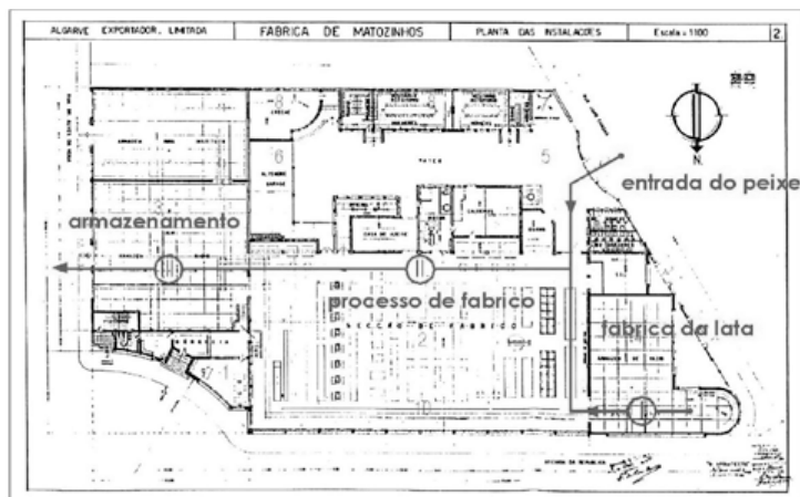
Fig. 6 – AEL: organização do espaço interno da fábrica segundo o projecto original de António Varela (Arquivo da CM de Matosinhos – a esquematização é nossa): verifica-se em planta a funcionalidade do sistema em cadeia que progride de forma linear, e de modo semelhante ao esquema apresentado no Quadro 1 (I: Secção de Vazio; II: Secção de Fabrico; III: Secção de Cheio) : a numeração representada corresponde à numeração da memória descritiva de António Varela: (1) gerência e acesso à habitação do encarregado; (2) secção de fabrico; (3) armazém de cheio; (4) armazém de vazio e depósito de sal; (5) entrada de serviço; (6) garagem; (7) depósito de água em elevação; (8) creche, vestiário, refeitórios e banheiros; (9) habitação do encarregado; (10) galeria na secção de fabrico. Em termos funcionais, é ainda possível observar a localização do núcleo constituído pela casa das caldeiras/motor/autoclaves, depósito de guano, chaminé, casa do azeite, oficina, garagem, pátio e armazém para instituto (fiscalização).
