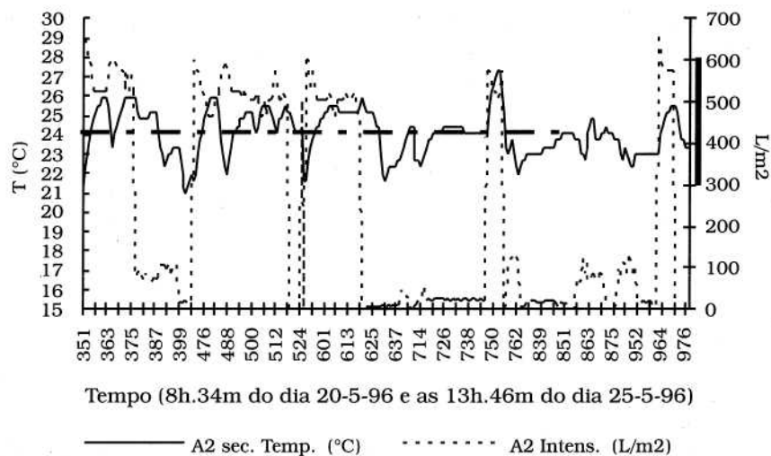
Fig. 16 - Luminosidade e Temperatura registadas na secretária do professor da sala 3.3 da FLUF? em períodos úteis do dia (entre as 8h34m do dia 20 de Maio de 1996 e as 13h46m do dia 25 de Maio de 1996).
