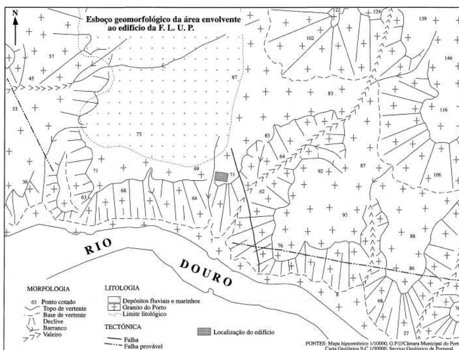
Fig. 5 - Esboço geomorfológico da área envolvente do novo edifício da FLUP (elaborado por Fátima Peixoto com a supervisão de Carmen Ferreira)
