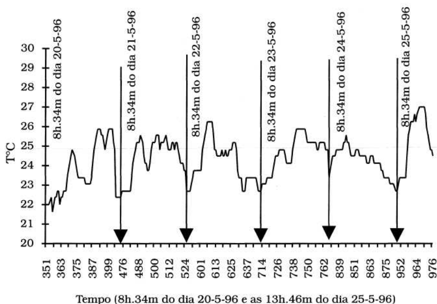
Fig. 13 - Temperatura registada no meio da sala 3.3 da FLUP em períodos úteis do dia (entre as 8h34m do dia 20 de Maio de 1996 e as 13h46m do dia 25 de Maio de 1996).
