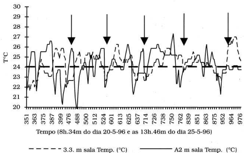
Fig. 14- Temperatura registada no meio das salas 3.3 e A.2, da FLUP? em períodos úteis do dia (entre as 8h34m do dia 20 de Maio de 1996 e as 13h46m do dia 25 de Maio de 1996).
