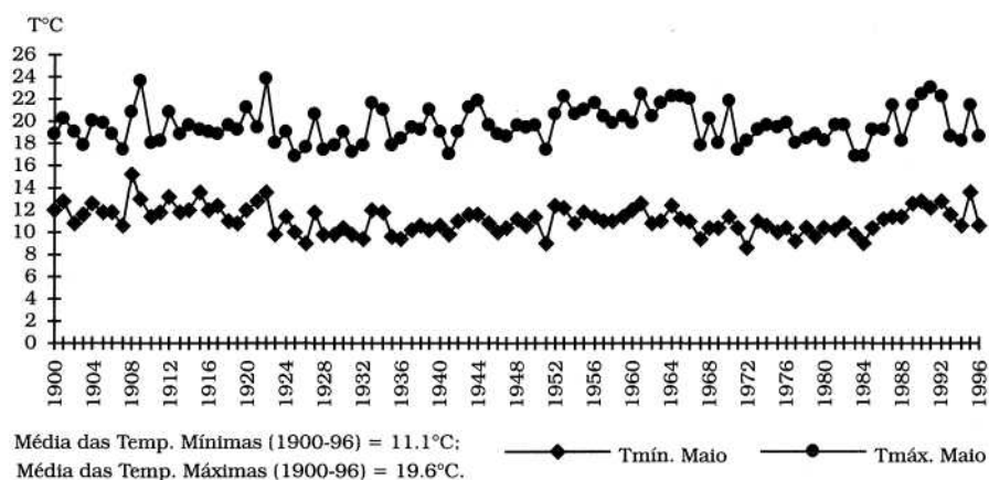
Fig. 9 - Temperatura média mensal mínima e máxima registada na estação de Porto-Serra do Pilar no mês de Maio entre 1900-96.
