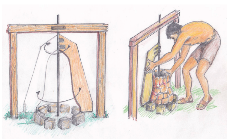
Fig. 13. Proceso de produción dos moldes da campá Fuente: M. A. Nieto Dorado
