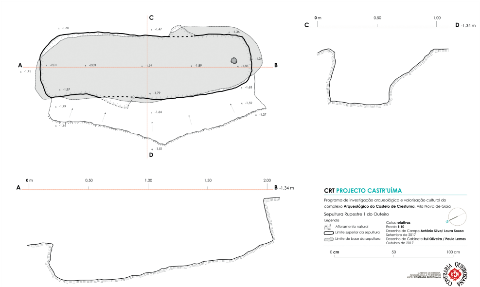
Fig. 9. Sepultura 1 do Outeiro: planta e secções axiais Fonte: A. Silva, L. Sousa, R. Oliveira e P. Lemos — Gabinete de História, Arqueologia e Património
