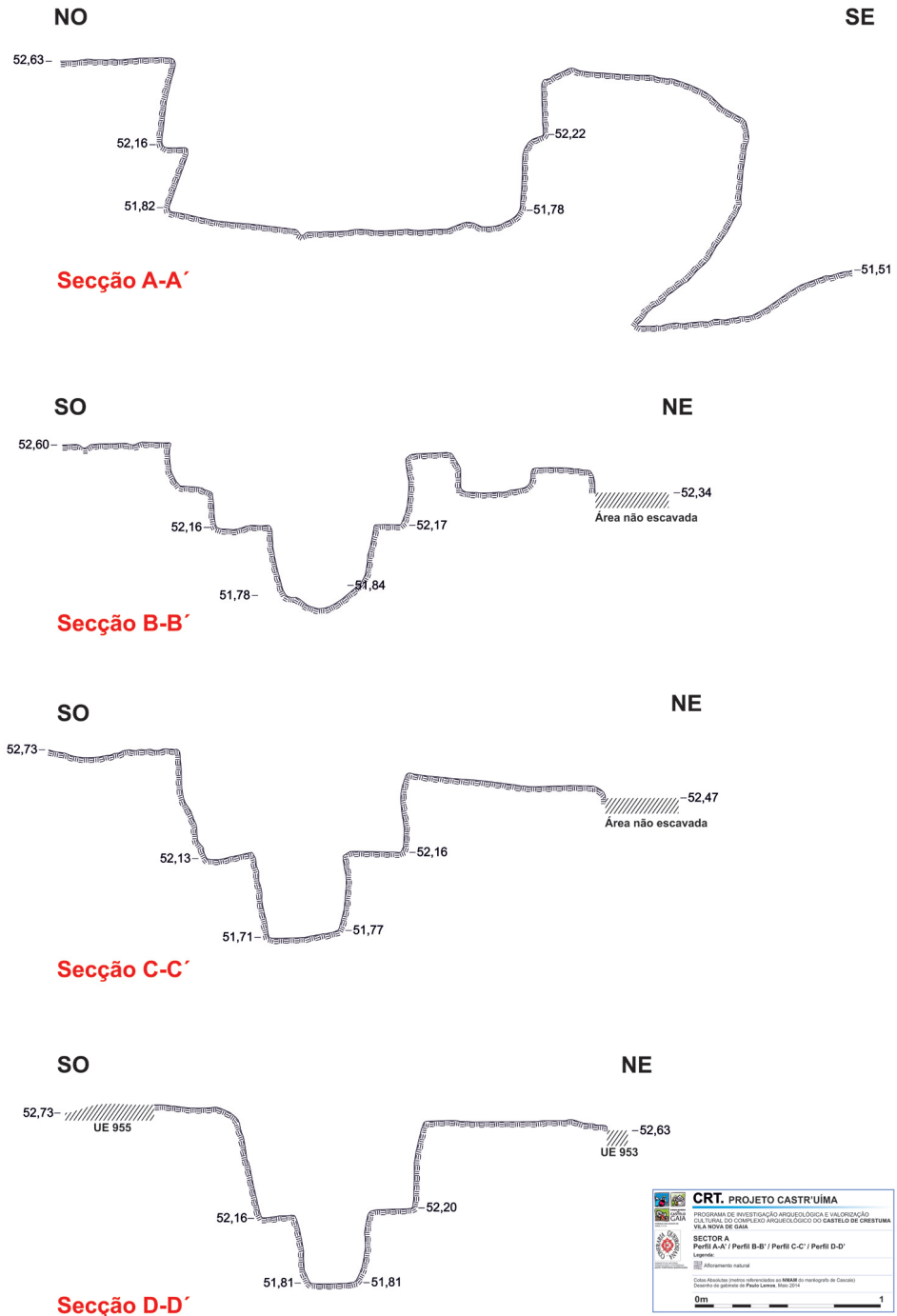
Fig. 7b. Sepultura 1 do Castelo: secção longitudinal e secções transversais Fonte: P. Lemos — Gabinete de História, Arqueologia e Património
