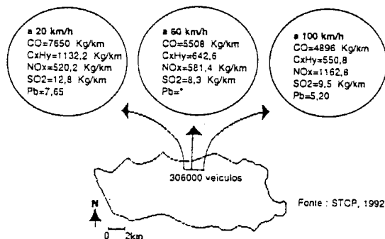
Fig.4 - Emissões prováveis para a atmosfera consoante a velocidade de circulação do número total de veículos que circulam diariamente no perímetro urbano portuense 5 (A. MONTEIRO, 1993).
