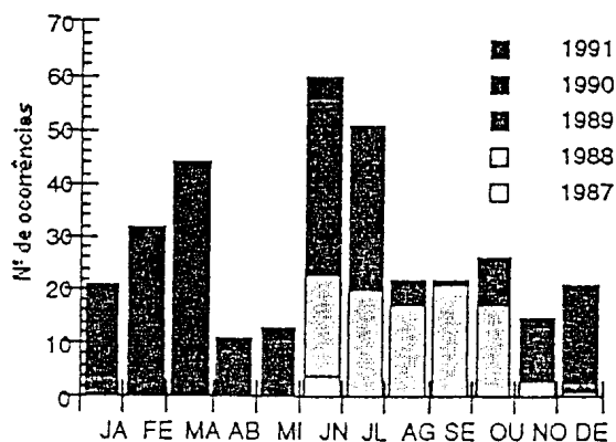
Fig.3 - Número de dias com \text{SO}_2 acima de 150 \mu\text{g}/\text{m}^3 nos postos da rede de avaliação da qualidade do ar da DGQA/Porto, localizados dentro ou próximo dos limites do concelho do Porto, entre 1 de Abril de 1987 e 31 Março de 1991 (A. MONTEIRO, 1993).
