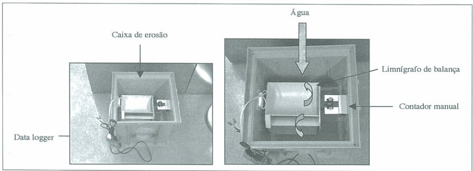
Fig. 20 | Limnígrafo de balança e data logger
